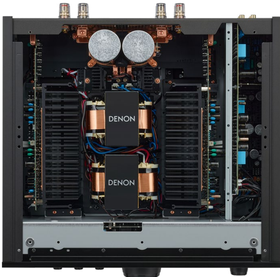
Schnörkel- aber auch kompromisslos: Das Design des PMA-3000NE zeugt von Erfahrung sowie anspruchsvoller Schaltungstopologie
