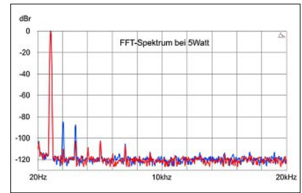
Das FFT-Spektrum des Vollverstärkers weist diesen als extrem „sauberen“ Kandidaten aus.
