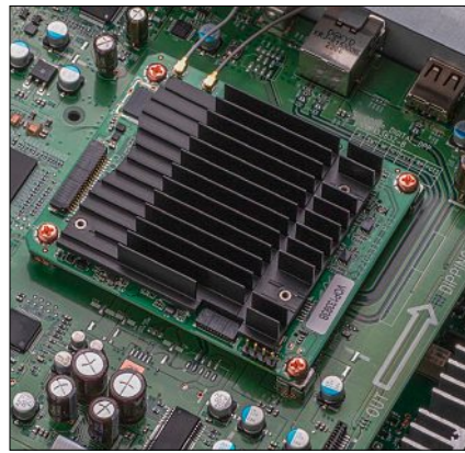
Hier befindet sich das „Hardware“-Herz der HEOS-Streaming- und Multiroom-Funktionalität.
