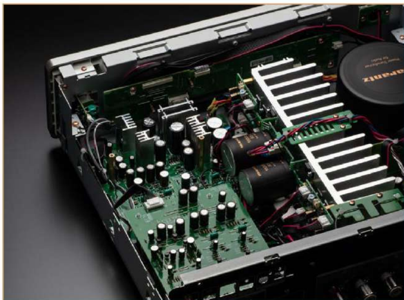
Unten links sehen wir das Phono-Board des Model 60n. Dieser Phono-Preamp ist für MM-Systeme ausgelegt und klingt mit diesen zusammen hervorragend
