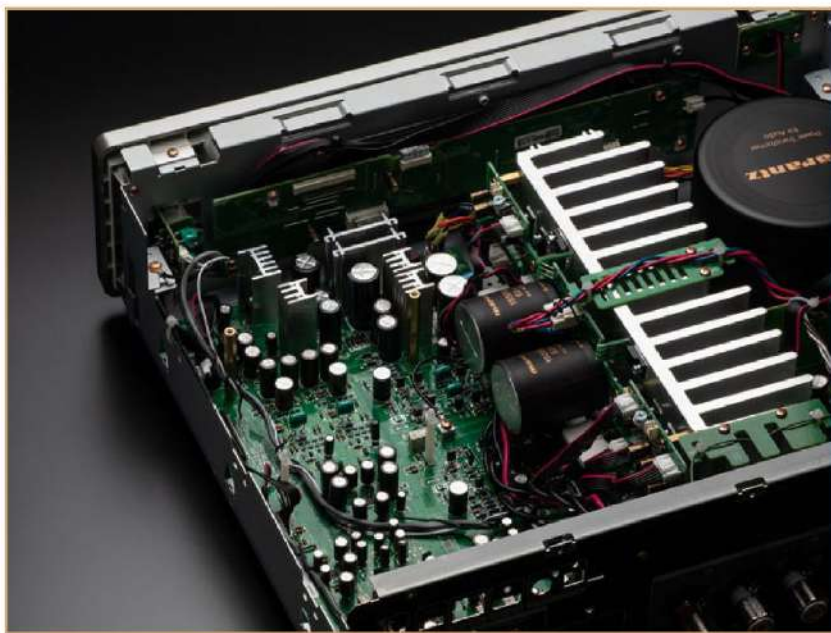
Hier im Bild sehen wir den Vorverstärker (links) und den Endverstärker (rechts) des Marantz Streaming-Amps
